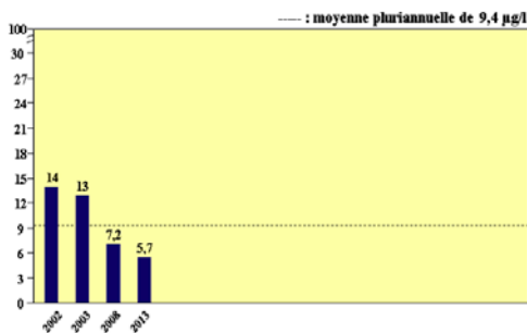
Concentrations estivales moyennes de phosphore (en haut) et de chlorophylle a (en bas) de 2002 à 2013 (µg/l)
